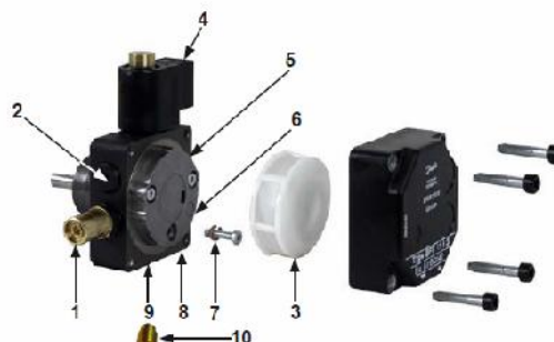
Cambio del filtro BFP 11
