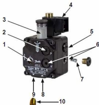
Cambio del filtro BFP 21
